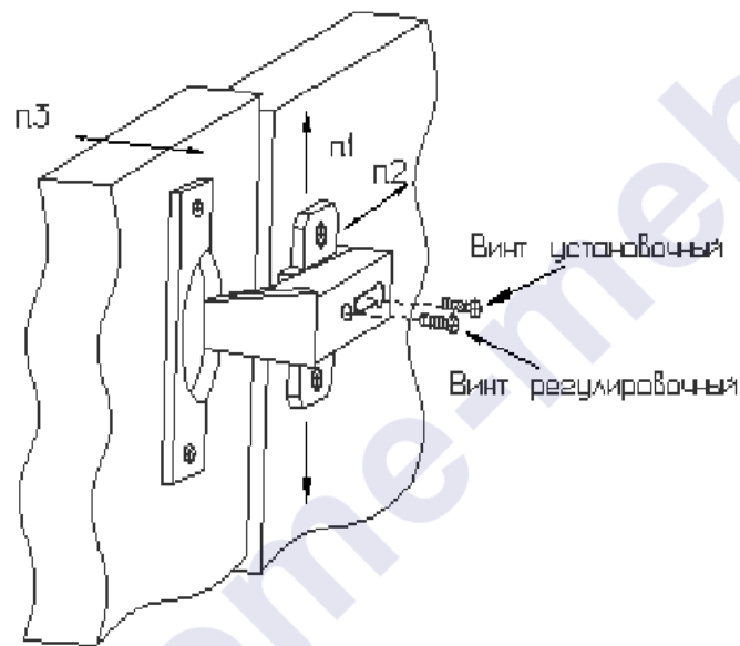
Установка фасадов.
