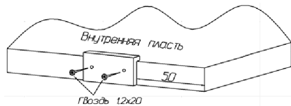
Рис.3. Установка подпятников.
